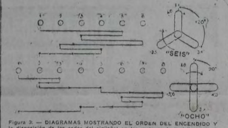
Figura 3. — DIAGRAMAS MOSTRANDO EL ORDEN DEL ENCENDIDO Y LA DISPOSICIÓN DE LOS CODOS DEL CIGÜEÑAL EN LOS MOTORES DE "SEIS" Y "OCHO" CILINDROS DEL TIPO "2-4-2".
