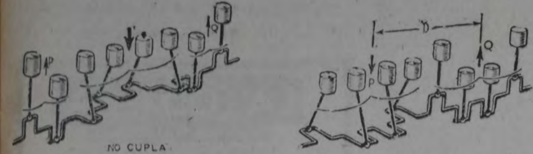
Figuras 1 y 2. — DOS FORMAS DE DISPONER LOS CODOS DE LOS CIGÜEÑALES DE LOS MOTORES DE OCHO CILINDROS EN LÍNEA (izquierda) El tipo "2-4-2", (derecha) el tipo "4-4". El primero o sea el tipo "2-4-2" da casi un equilibrio perfecto, pues las fuerzas secundarias P y Q equilibran a la fuerza resultante R. En el tipo "4-4" las fuerzas secundarias P y Q generan una "cupla" tendiente a mecer o trepidar el motor.
